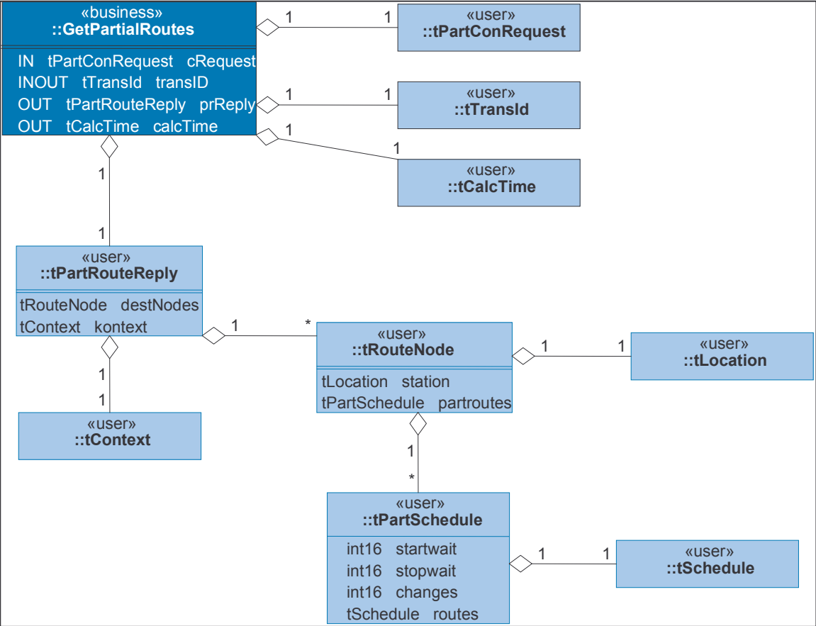
Abbildung: Struktur der Methode GetPartialRoutes des Interfaces DistributedScheduleInfo
