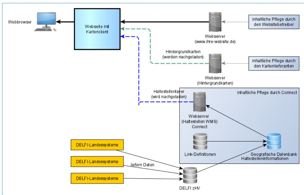
[Bild 1] Schemadarstellung der beteiligten Services
